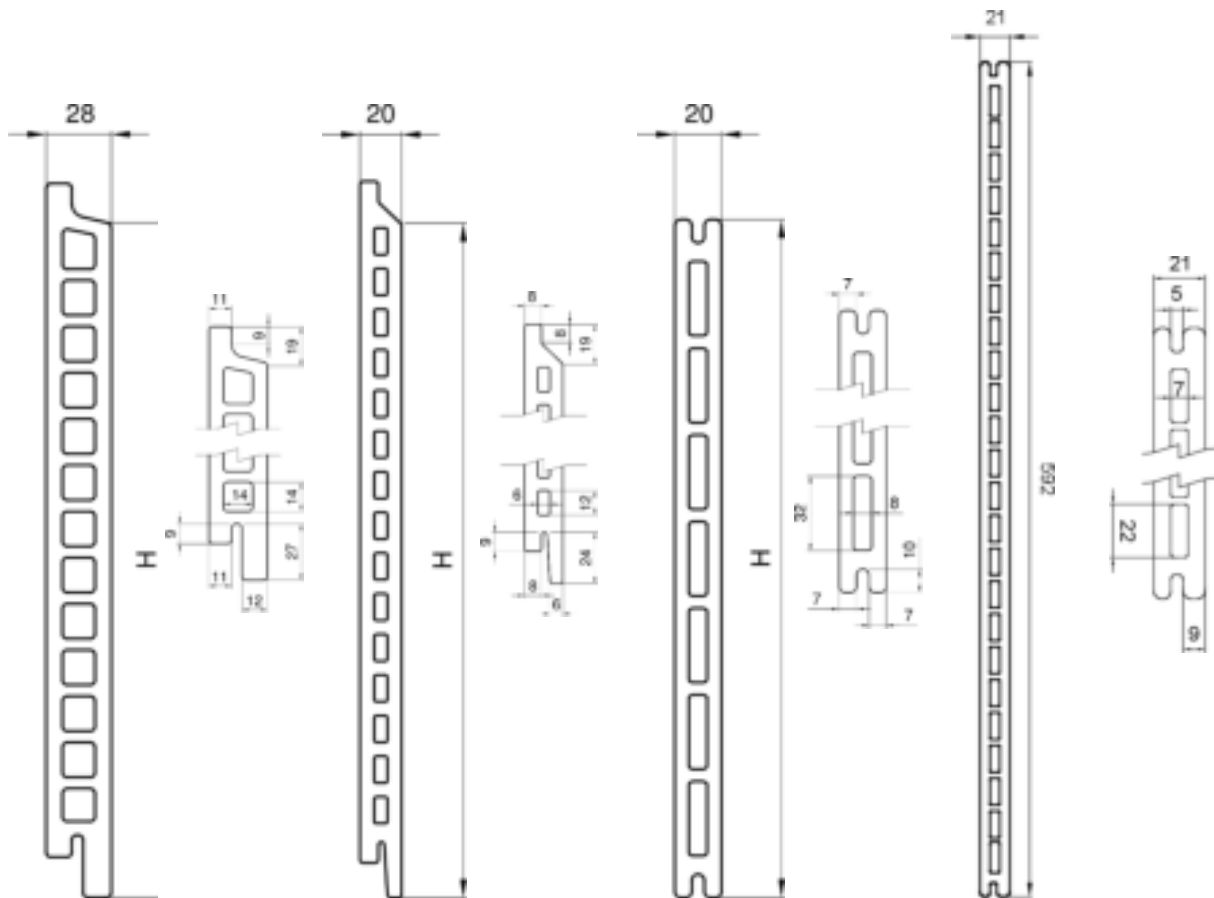
Figure A1.1a: Faveton® Ceram 28.
